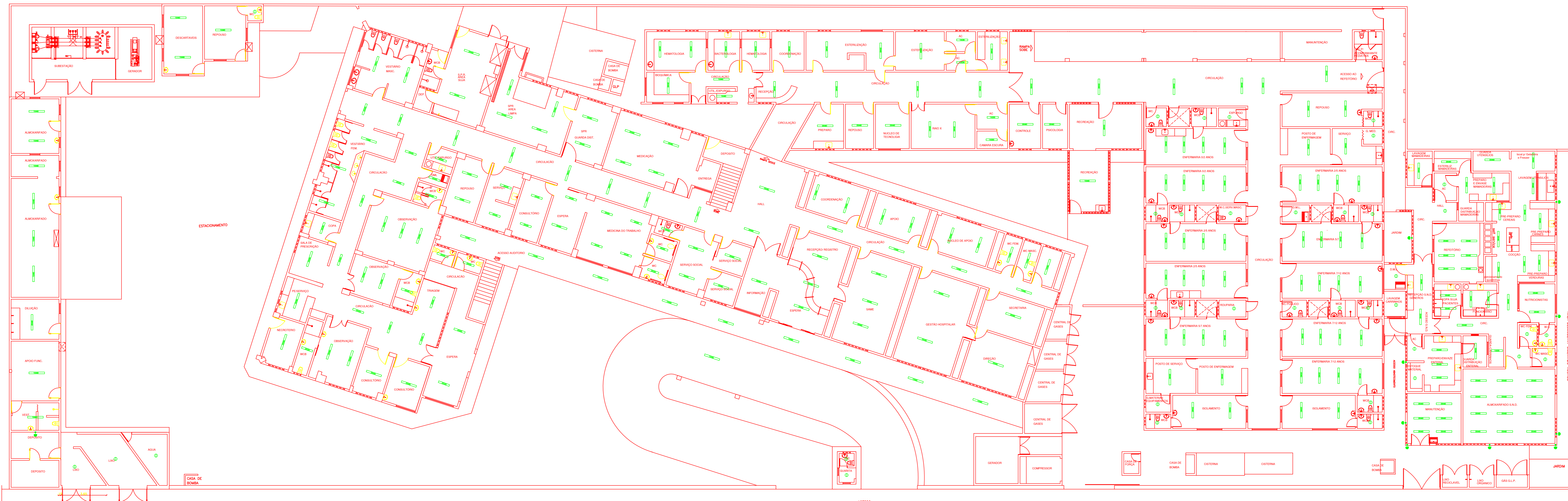
PLANTA BAIXA PAVTO. TERREO ESCALA 1/100
