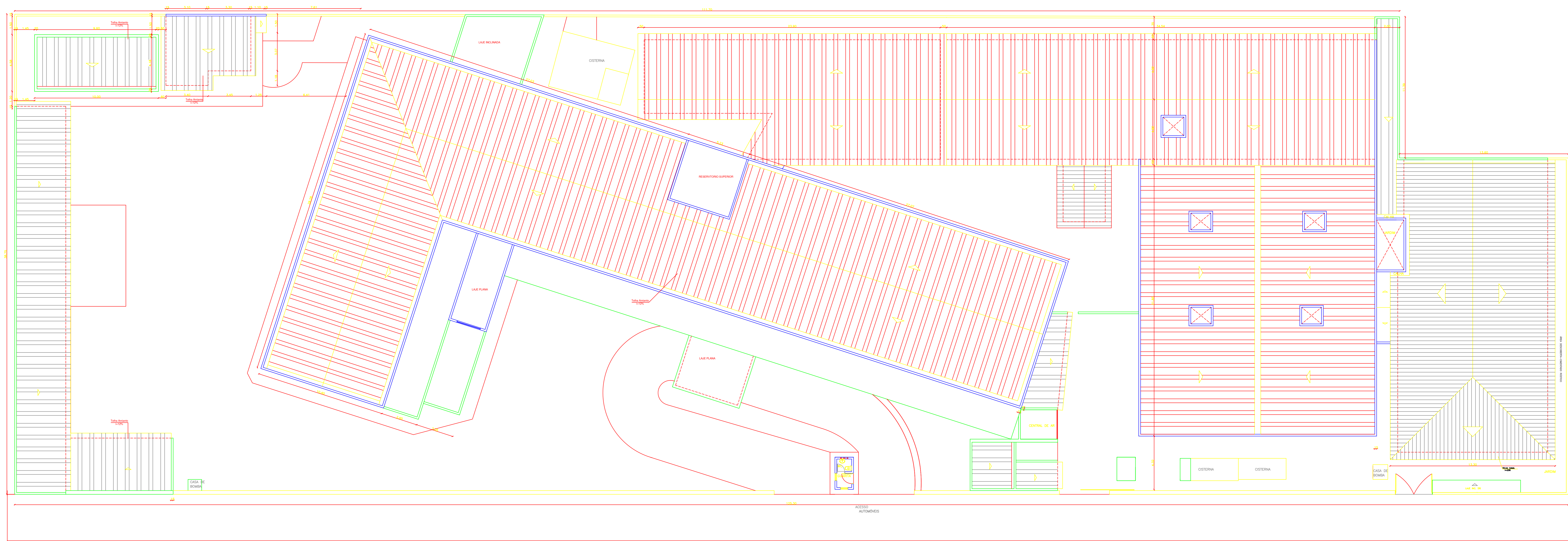
PLANTA DE COBERTA ESCALA 1/100
